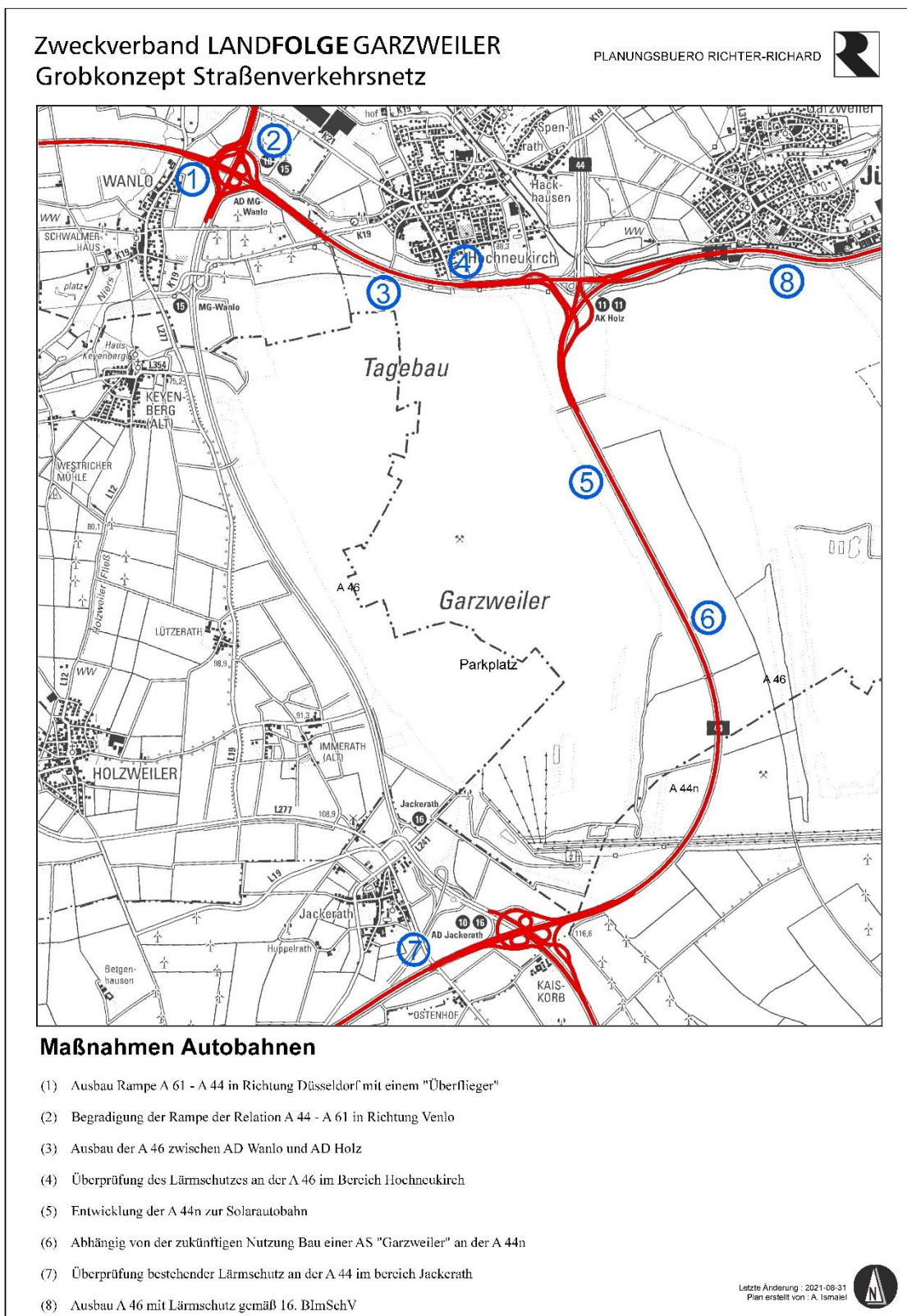
Abb. 4.1: Optimierungsmaßnahmen Autobahnen
