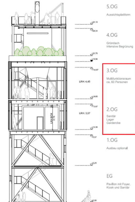
Grundriss 2. & 3.Obergeschoss Querschnitt
